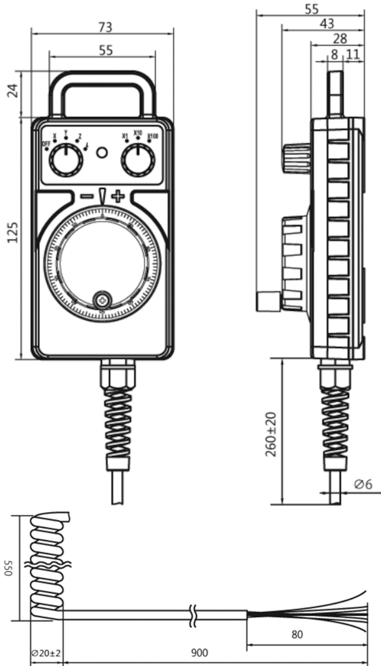
DC2手持盒 产品尺寸平面图
